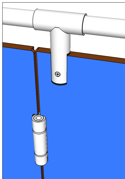
Pinza fissaggio superiore e tubo acciaio Inox
